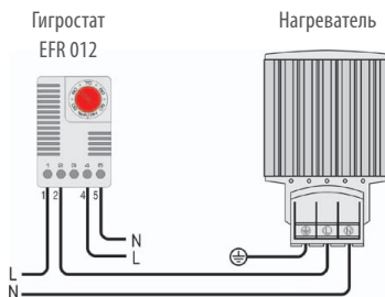
Пример подключения
