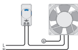
Термостат STS 011 (NO) Напр., вентилятор
