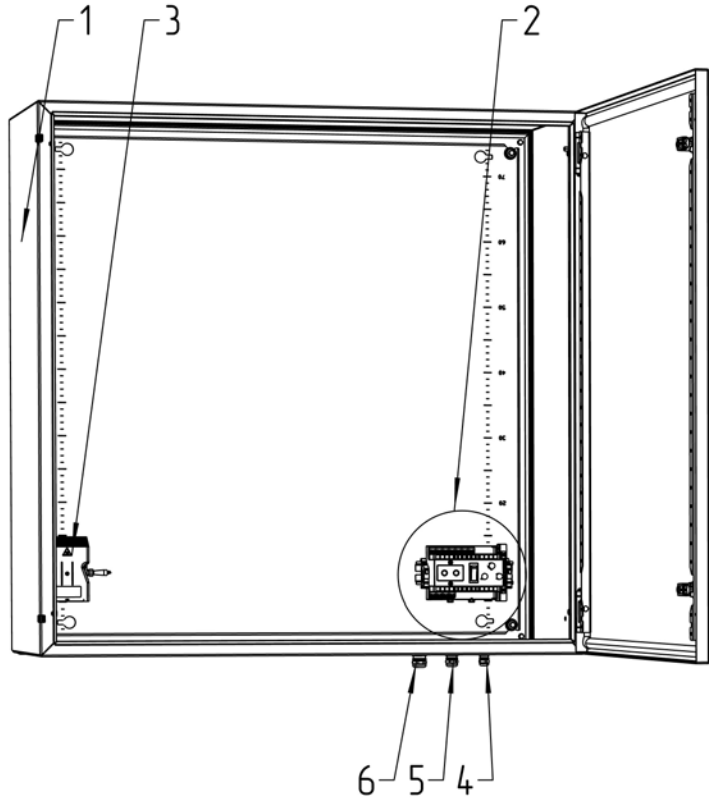
Расположение оборудования на DIN-рейке М 1:3
