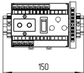
Расположение оборудования на DIN-рейке М 1:3
