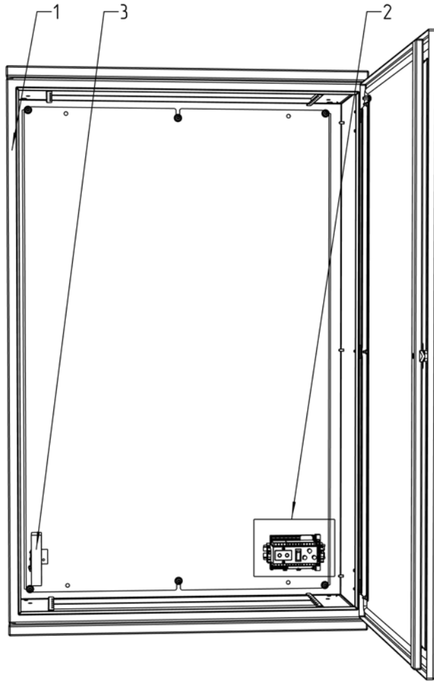
Расположение оборудования на DIN-рейке М 1:3
