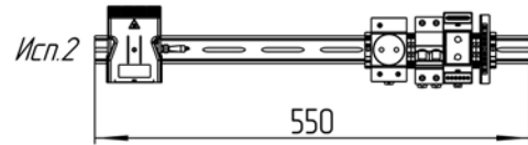
Расположение оборудования на DIN-рейке М 1:3
