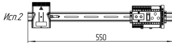
Расположение оборудования на DIN-рейке М 1:3
