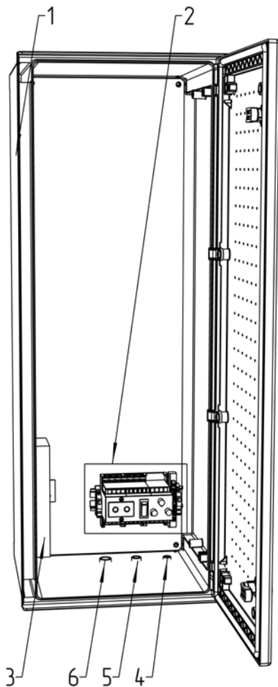
Расположение оборудования на DIN-рейке М 1:3
