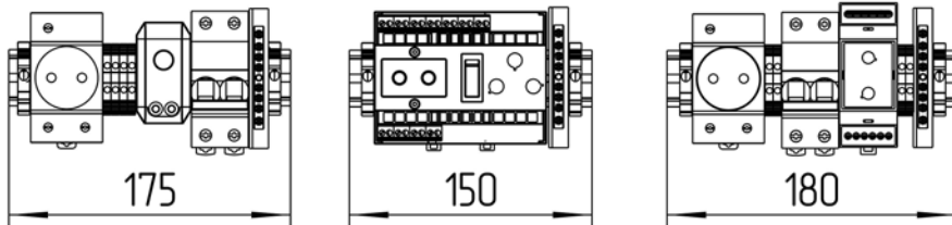
Расположение оборудования на DIN-рейке М 1:3
