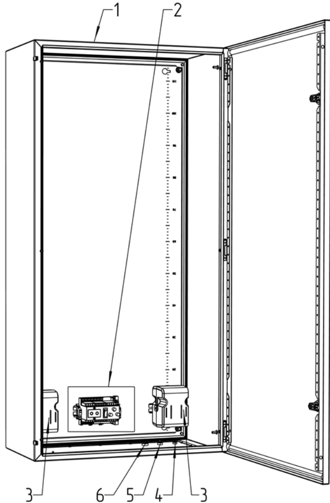
Расположение оборудования на DIN-рейке М 1:3
