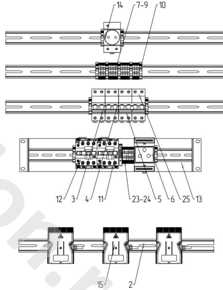
Расположение оборудования на DIN-рейке М 1:3
