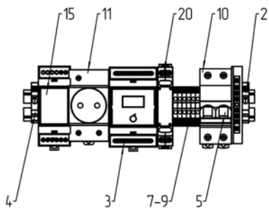
Расположение оборудования на DIN-рейке
